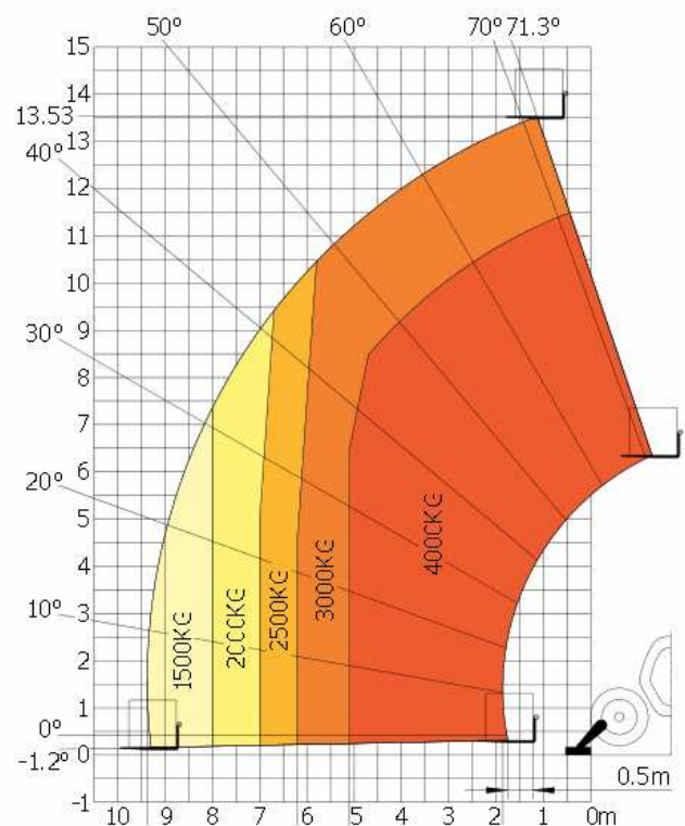
Ábaco de carga (EN1459-B) com estabilizadores :
